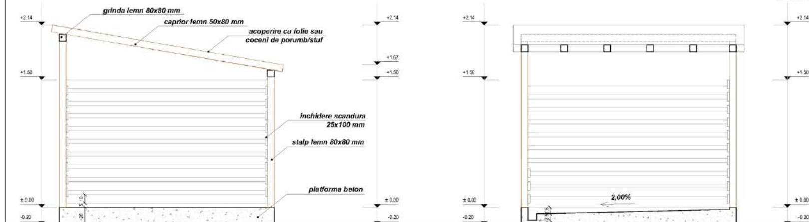
SECTIUNE AA' SC. 1:25
